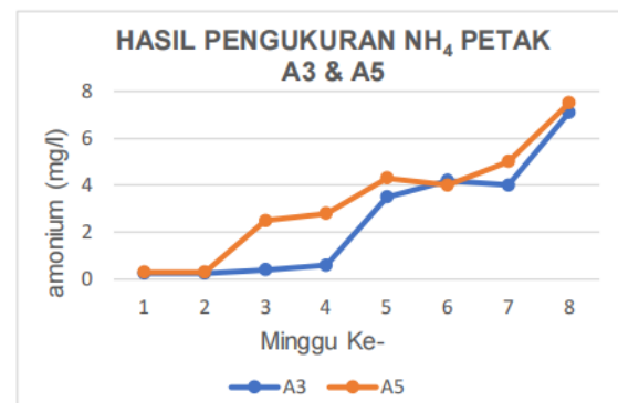
Gambar 4. Hasil Pengukuran \text{NH}_4 pada Petak A3 dan A5
