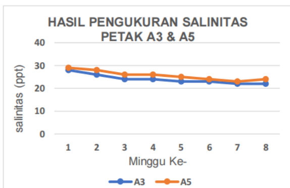
Gambar 2. Hasil Pengukuran Salinitas pada Petak A3 dan A5
