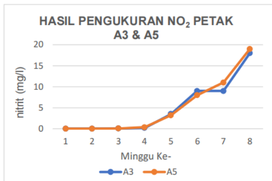
Gambar 6. Hasil Pengukuran \text{NO}_2 pada Petak A3 dan A5
