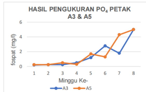
Gambar 7. Hasil Pengukuran \text{PO}_4 pada Petak A3 dan A5
